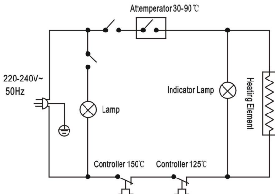
BZ-CTH97/BZ-CTH107/BZ-CTH137
