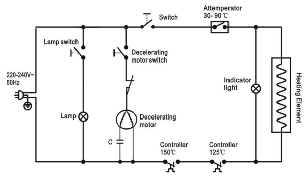
BZ-CTH97-2
