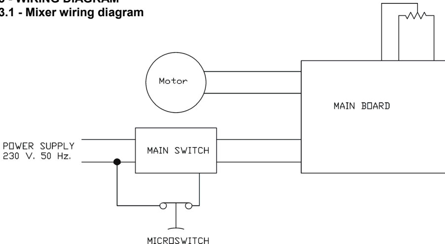
FIG. n. 5 - Wiring diagram
