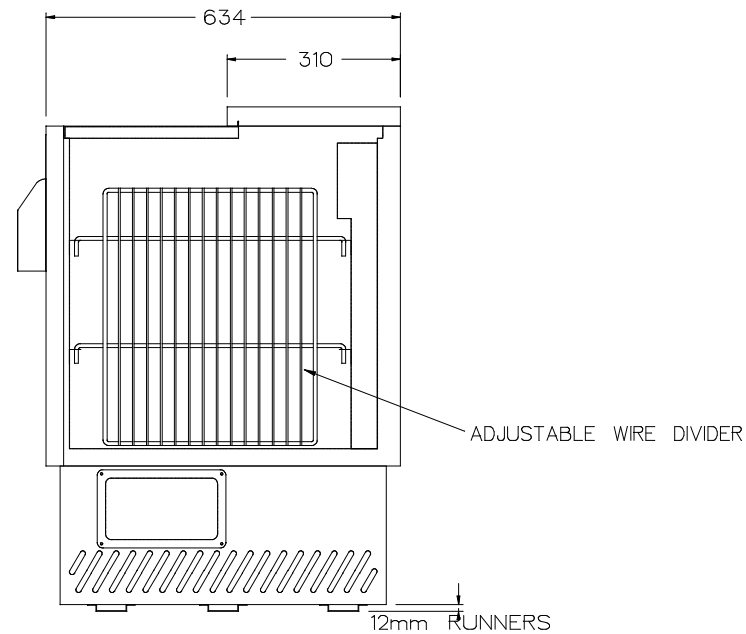
END ELEVATION
