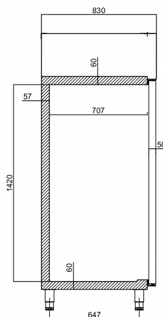
A-A
